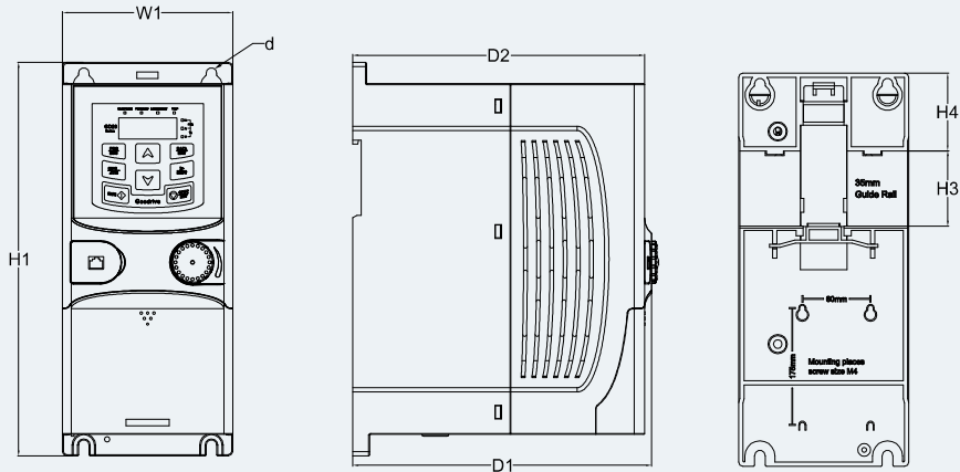
Установочные размеры (мм)
