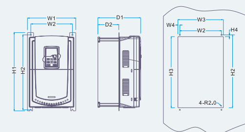
Фланцевый монтаж преобразователей 11 ~ 15кВт
