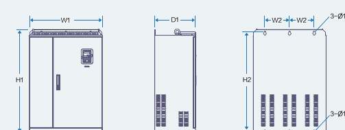
Настенный монтаж преобразователей 220 ~ 350кВт
