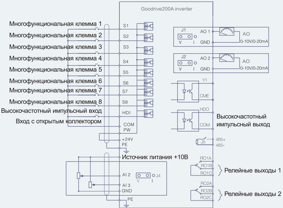
Схема подключения цепи управления
