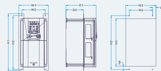
Фланцевый монтаж преобразователей 18,5 ~ 30кВт
