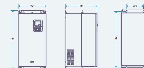
Фланцевый монтаж преобразователей 132 ~ 200кВт
