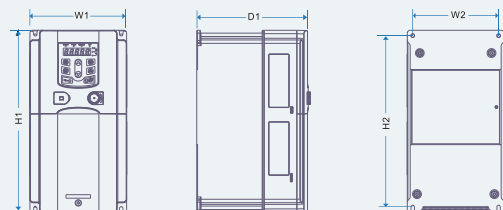
Схема установки для ПЧ 11—15кВт
