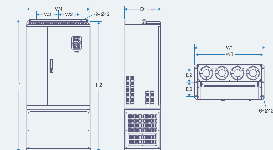
Напольный монтаж преобразователей 350—500кВт
