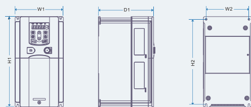
Настенный монтаж преобразователей 18,5 ~ 30кВт
