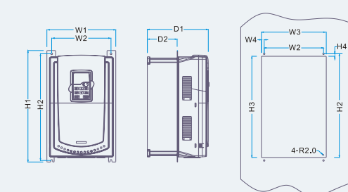
Фланцевый монтаж преобразователей 37 ~ 110кВт
