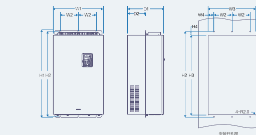
Фланцевый монтаж преобразователей 132 ~ 200кВт
