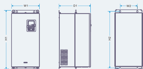
Схема установки для ПЧ 18—55кВт
