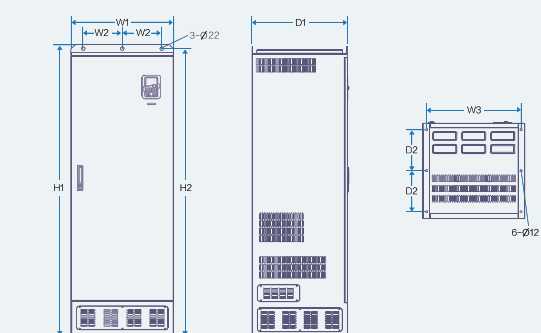
Напольный монтаж преобразователей 350—500кВт
